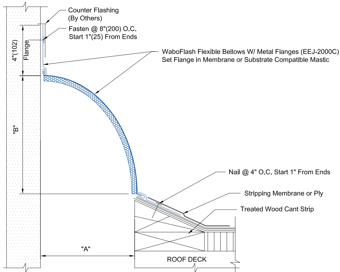
EEJ/C-2000 DETAIL
