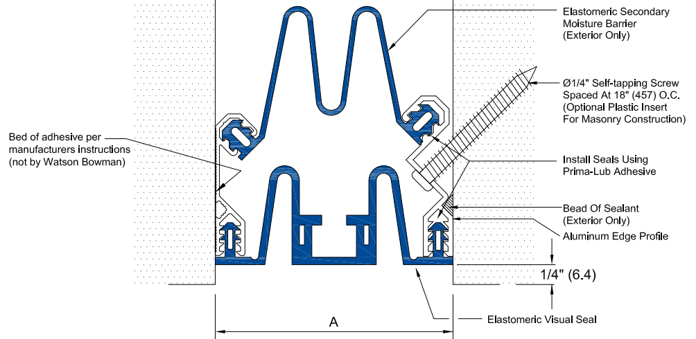
WSC-300 DETAIL
